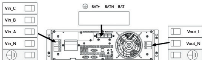
Рис. слева (снизу вверх): Заземление (GND), вход N, вход A(L1), вход B(L2), вход C(L3); Рис. в середине (слева направо): Заземление (GND), аккумуляторные батареи BAT+, BAT N, BAT-; Рис. справа (снизу вверх): Заземление (GND), выход N, выход L.
